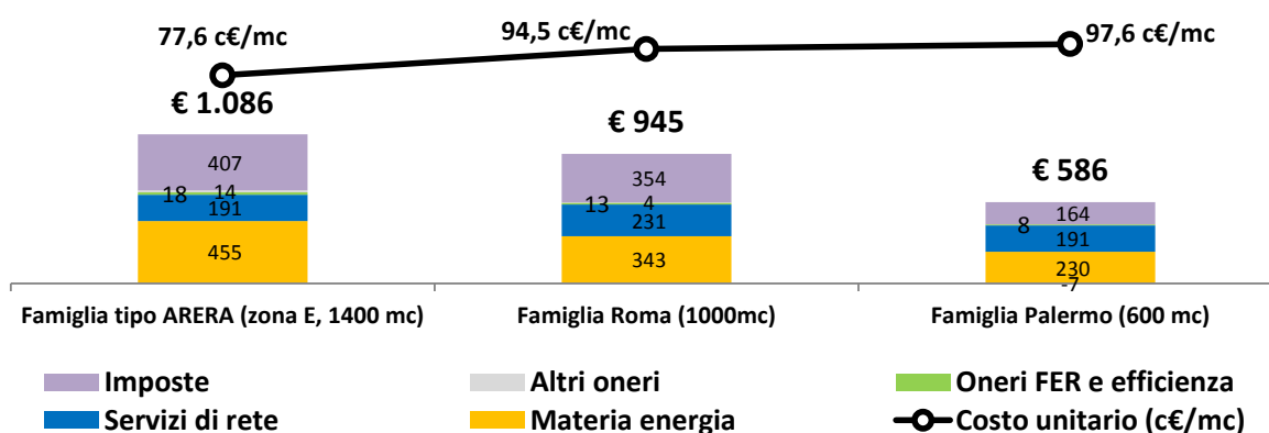
Confronto bolletta gas tra famiglie residenti in diverse zone climatiche
