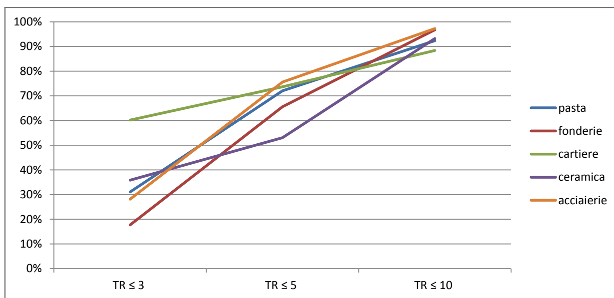
Figura A.2 - Analisi degli investimenti necessari per gli interventi, per comparto e tempo di ritorno (TR)
